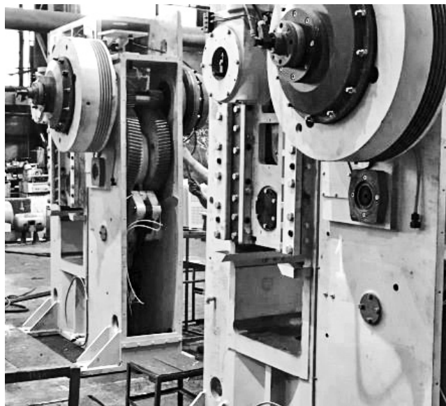
Чеканочный пресс для изготовления орденов и медалей.
